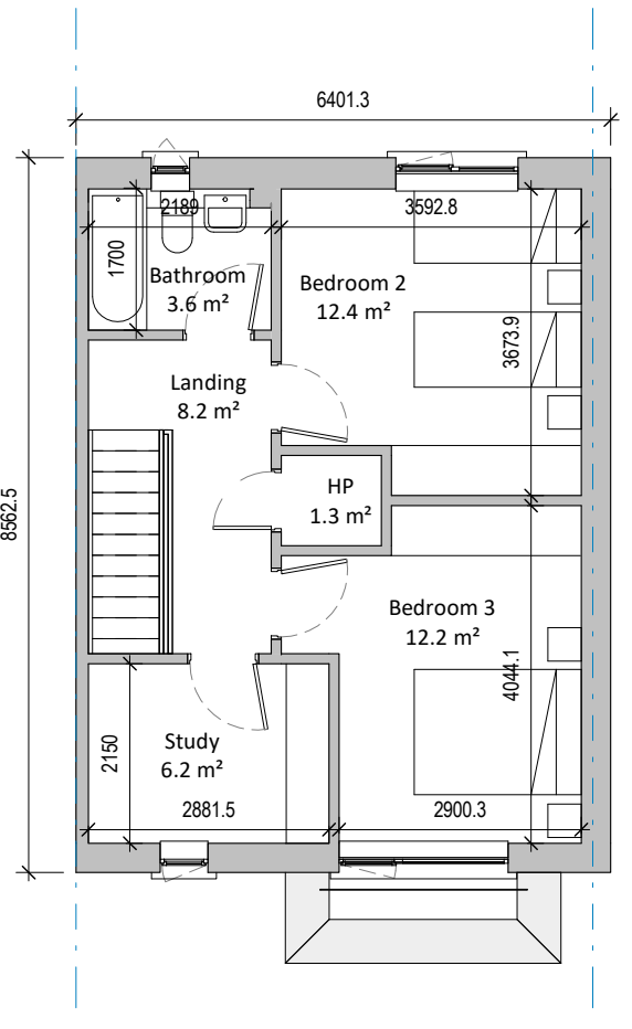
4 H08R Level 02 1 : 100
