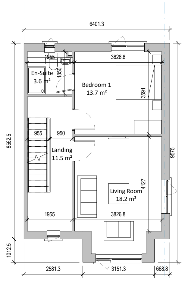
3 H08R Level 01 1 : 100
